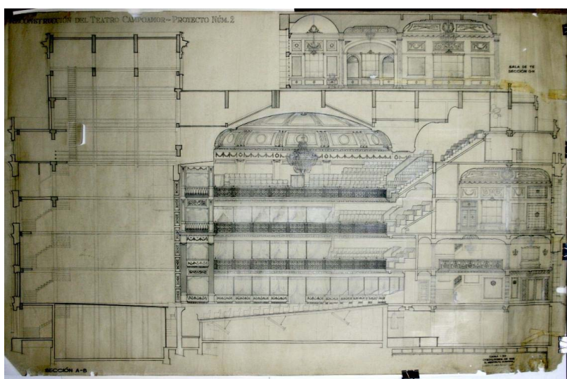
Plano de Gabriel de la Torriente del Proyecto nº 2 de reconstrucción del Teatro Campoamor. 1942
